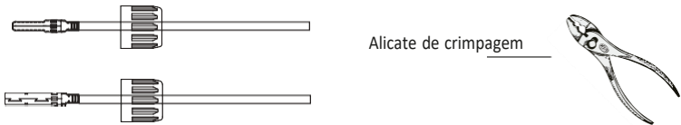
Fig5.4 Prenda o pino de contato ao fio
