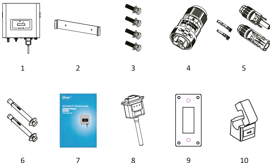
Fig1.3 Desenho dos acessórios
