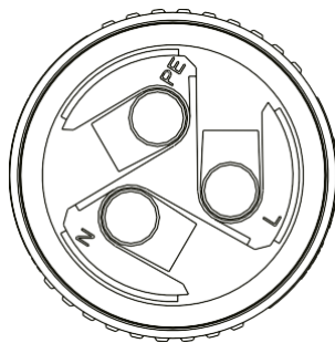
Fig5.9 Padrão do furo do conector CA
